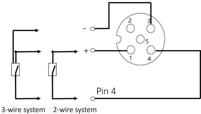
PNP input
