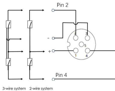
PNP input
