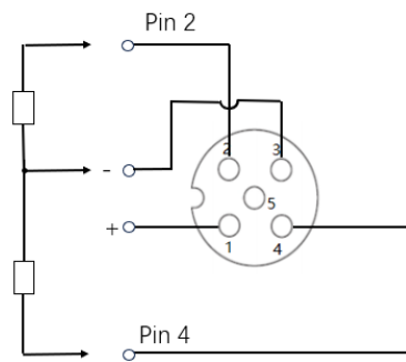
PNP output
