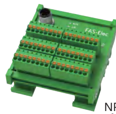
NPN 전환가능
